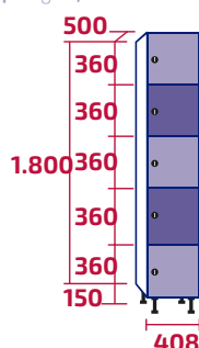
AMP400/1 COD: 10460 | 10509 44kg | 47kg · 0,37m 3
