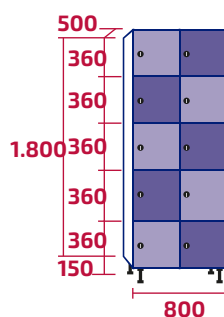
AMP400/2 COD: 10461 | 10510 79kg | 85kg · 0,72m 3
