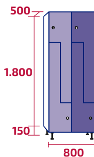
AML400/2 COD: 10531 79kg · 0,71m 3
