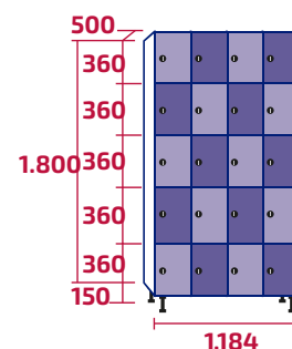
AMP300/4 COD: 10459 | 10508 126kg | 135kg · 1,07m 3
