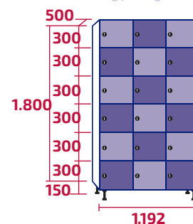
AMB400/3 COD: 10469 | 10518 122kg | 130kg · 1,07m 3
