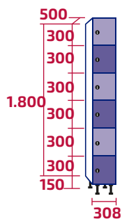
AMB300/1 COD: 10463 | 10512 41kg | 43kg · 0,28m 3
