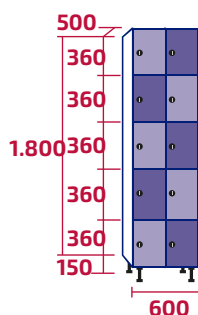
AMP300/2 COD: 10457 | 10506 68kg | 72kg · 0,54m 3
