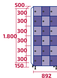
AMB300/3 COD: 10465 | 10514 103kg | 110kg · 0,80m 3
