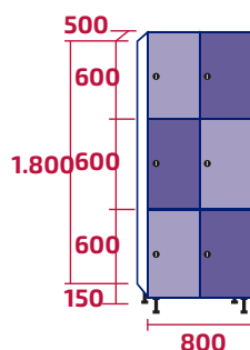
AMM400/2 COD: 10447 | 10496 68kg | 74kg - 0,72m 3
