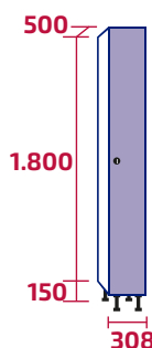
AMV300/1 COD: 10428 | 10477 32kg | 34kg · 0,28m 3
