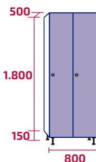
AMV400/2 COD: 10433 | 10482 62kg | 68kg · 0,72m 3
