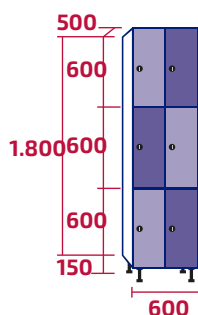
AMM300/2 COD: 10443 | 10492 60kg | 64kg - 0,54m 3
