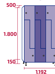
AML400/3 COD: 10532 113kg · 1,05m 3
