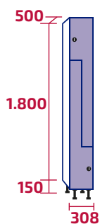
AML300/1 COD: 10526 40kg · 0,28m 3
