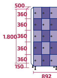
AMP300/3 COD: 10458 | 10507 97kg | 104kg · 0,80m 3
