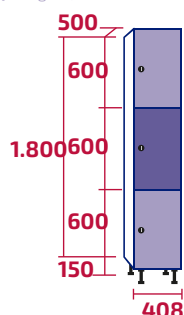
AMM400/1 COD: 10446 | 10495 39kg | 42kg - 0,37m 3
