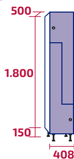
AML400/1 COD: 10530 44kg · 0,36m 3
