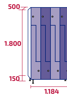
AML300/4 COD: 10529 129kg · 1,07m 3
