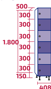
AMB400/1 COD: 10467 | 10516 47kg | 50kg · 0,37m 3
