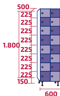
AMZ300/2 COD: 10471 | 10520 81kg | 85kg · 0,54m 3
