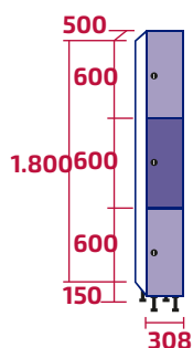
AMM300/1 COD: 10442 | 10491 35kg | 37kg - 0,28m 3
