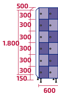
AMB300/2 COD: 10464 | 10513 72kg | 77kg · 0,54m 3
