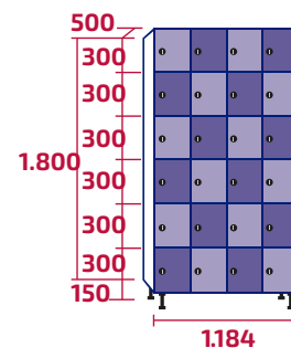
AMB300/4 COD: 10466 | 10515 135kg | 144kg · 1,07m 3
