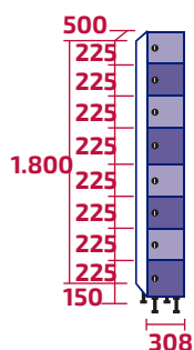
AMZ300/1 COD: 10470 | 10519 45kg | 47kg · 0,28m 3
