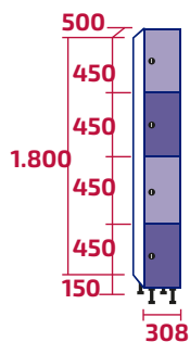
AMC300/1 COD: 10449 | 10498 37kg | 39kg - 0,28m 3
