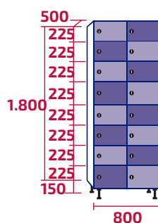
AMZ400/2 COD: 10475 | 10524 94kg | 100kg · 0,72m 3
